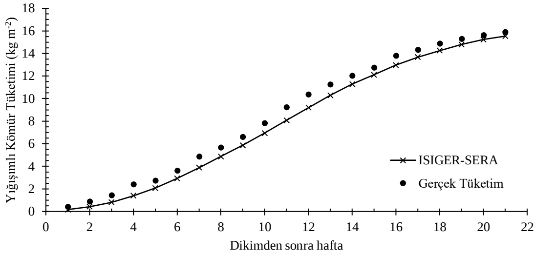
Şekil 4. Adana iklim koşullarında ısı perdeli PE plastik serada üretim periyodu boyunca tüketilen ve ISIGER-SERA modeline göre hesaplanan yığılmış kömür miktarı (kg m⁻²)
